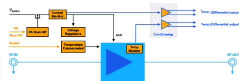
内部ブロック図
