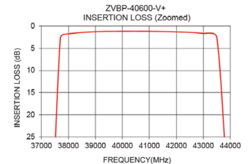
ZVBP-40600-V+ 37700~43500MHz Case Style UH3130 80 x 16 x 8.1 mm (コネクタ部、突起部含まず)
