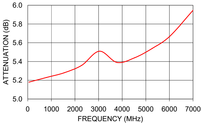
PAT-5+ ATTENUATION
