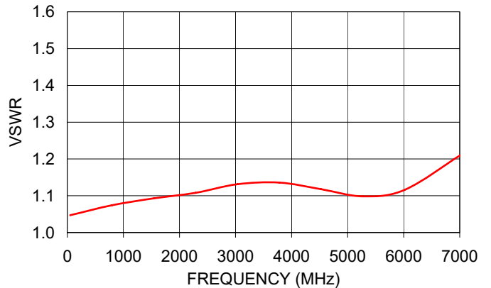
PAT-5+ VSWR
