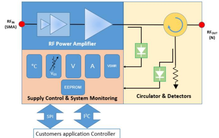
ZHL-2425-250+ 内部ブロック図
